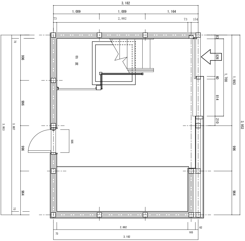
一階平面圖 1/30
