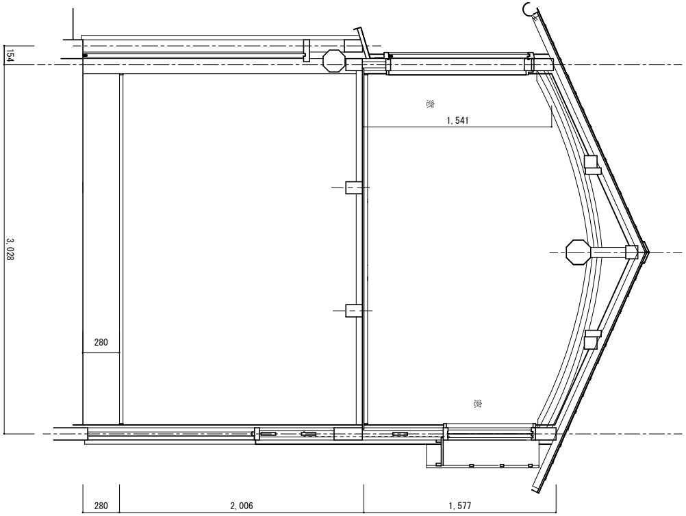
北側断面図 1/30
