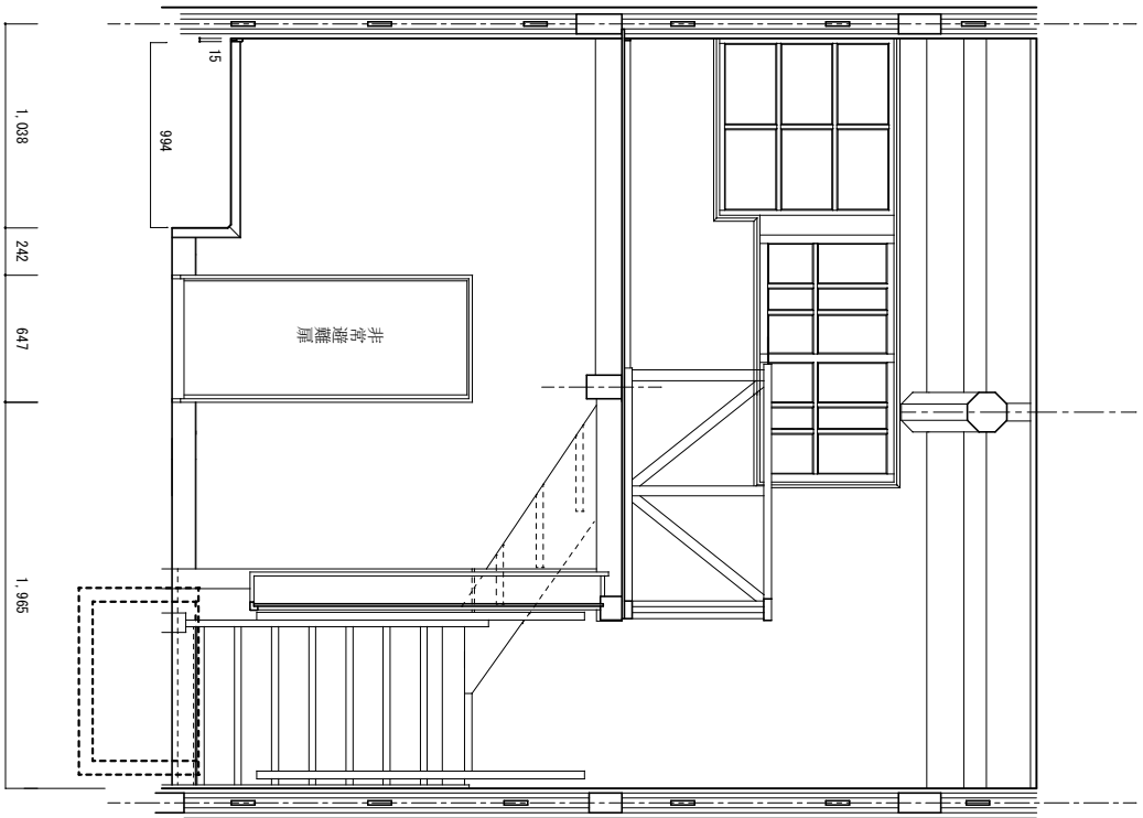
東側断面図 1/30
